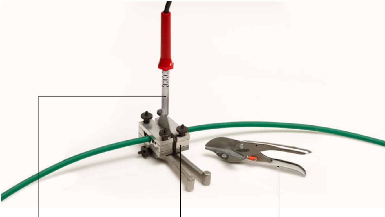
Schweißkolben mit teflonisiertem Schweißspiegel Soldering iron with teflon-coated welding tip
